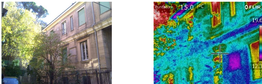
Figura.3 – Rilievo termografico del prospetto Nord – 3
