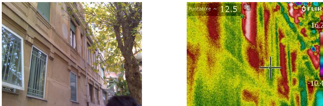
Figura.4 – Rilievo termografico dei serramenti esterni prospetto Sud
